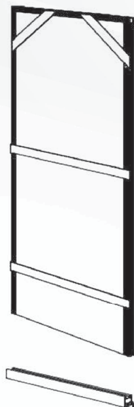
1x Perfil cabecero 2x Perfil vertical
